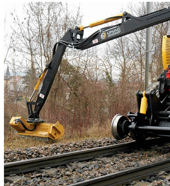
Obr.: Lesní fréza typu BMS F na dvojcestném rýpadle.
