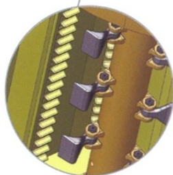
Rotor s kladívky SMO a protiřezy (sériově u H-SMO-B)
